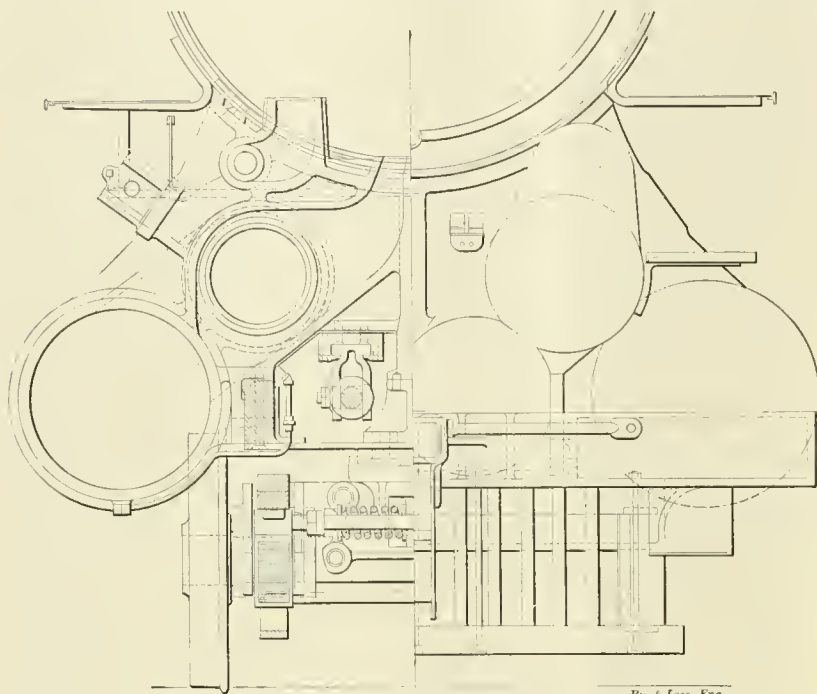
SECTION OF 4-CYLINDER COMPOUND, N. Y. C. & H. R. R.
